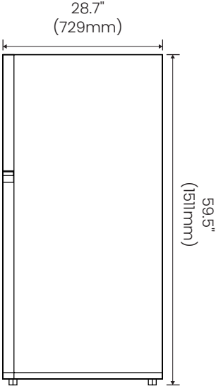
Vue droite
